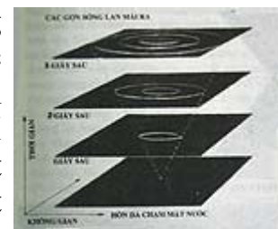
Hình 2.3: vòng tròn lớn dần của các gợn sóng sẽ tạo thành một nón có đỉnh nằm đúng tại chỗ và tại thời điểm hòn đá chạm vào mặt nước.
