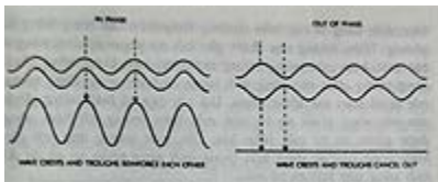
Hình 4.1: Nếu đỉnh của tập hợp sóng này trùng với hõm của tập hợp sóng kia, thì chúng sẽ triệt tiêu lẫn nhau chứ không cộng lại để trở thành mạnh hơn.
