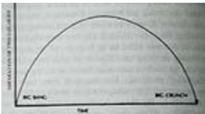
Hình 3.2: Khoảng cách giữa hai thiên hà lân cận thay đổi từ 0, tăng tới cực đại rồi lại giảm dần xuống 0.
