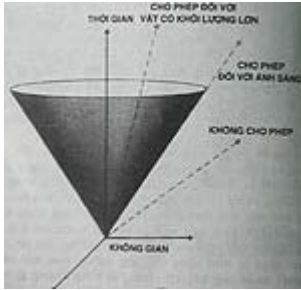
Hình 2.7: Nón ánh sáng của các sự kiện trên đường đi của vật thể trong không gian.
