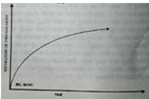
Hình 3.4: Sự tách biệt giữa hai thiên hà cũng bắt đầu từ 0 và tăng lên mãi mãi.
