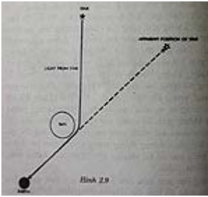
Hình 2.9: Điều này có nghĩa là ánh sáng từ một ngôi sao xa khi đi qua gần mặt trời có thể bị lệch đi một góc nhỏ.
