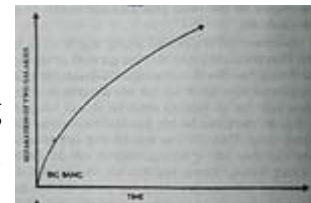
Hình 3.3: Hai thiên hà ngày càng tách xa nhau.
