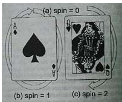
Hình 5.1 a, b, c: Hình minh họa về các dạng spin khác nhau của hạt.
