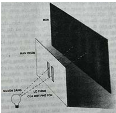
Hình 4.2: Chỉ có một lượng sáng nhỏ đi qua khe.
