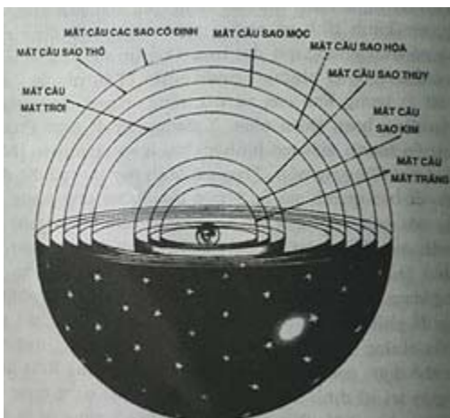
Hình 1.1: Mô hình vũ trụ của Aristotle - Ptolemy coi trái đất là trung tâm của vũ trụ.
