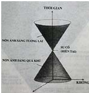
Hình 2.4: Mặt nón ánh sáng quá khứ là tập hợp các sự kiện mà từ chúng một xung ánh sáng có thể tới được sự kiện đang xét.
